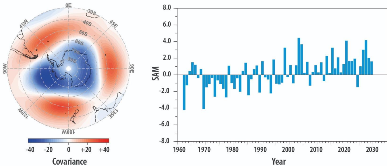
Fig. 2 : Structure et évolution temporelle du SAM ( Southern Annular Mode ), principal mode de variabilité de l'atmosphère extra-tropicale de l'hémisphère Sud : (a) amplitude des anomalies de pression atmosphérique à 500 hPa liées au SAM ; (b) indice du SAM sur la période 1957-2024. La phase positive du SAM (indice de SAM > 0) correspond à des anomalies de pression négatives autour du continent antarctique et positives dans les latitudes tempérées (au nord de 60°S) résultant dans une intensification et une migration vers le sud des vents d'ouest. Source: Wachter et coll., 2020 ; NERC-BAS An observation-based Southern Hemisphere Annular Mode Index.
